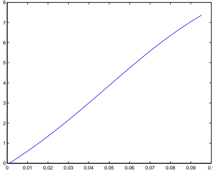
Fig. 11. \|u^\varepsilon\|_{L^2(O_\varepsilon)} = f(\varepsilon)
